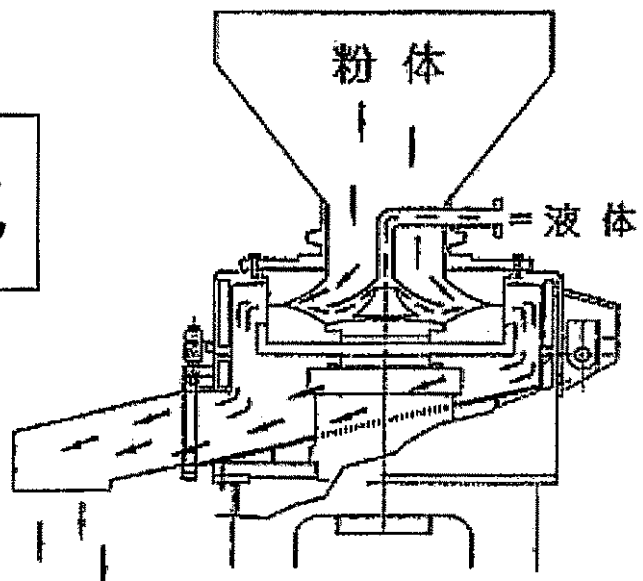
粉碎室で液体と粉体が連続混合
