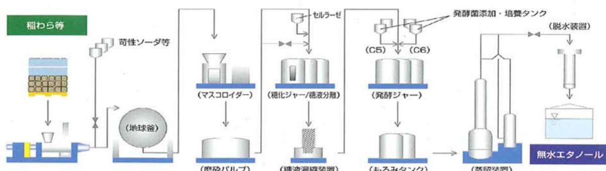
図 1-4. プラントの概念図
