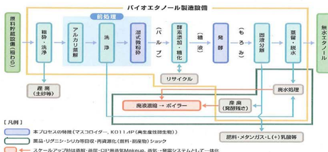
図 1-3. バイオ燃料製造モデルプラントフロー
