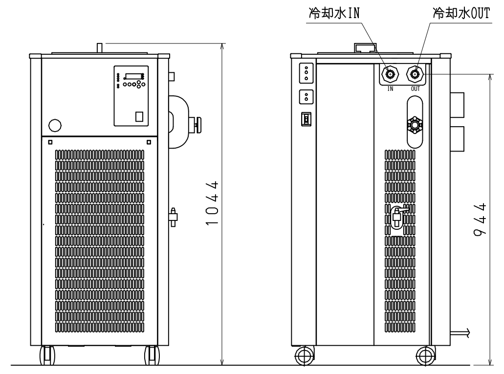
冷却水循環装置
